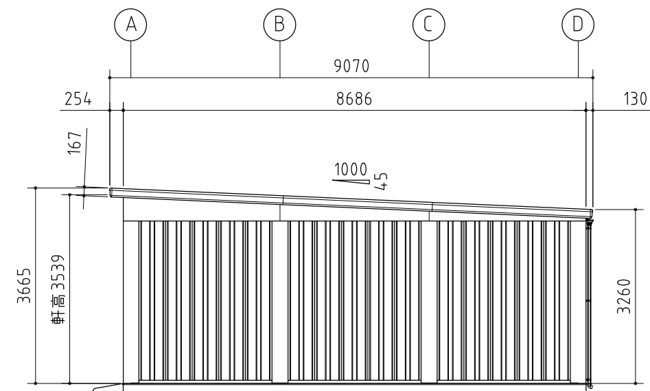
側面図
