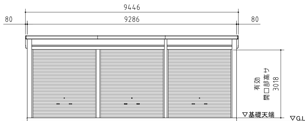
正面図
